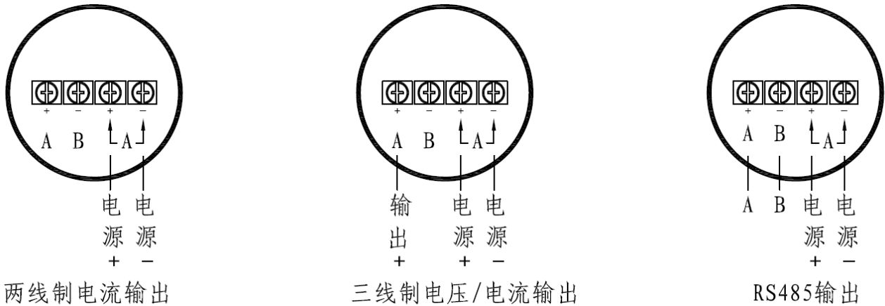
图一: 接线图
