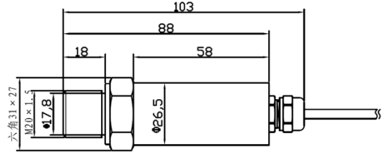
图二: 直接出线引出形式
