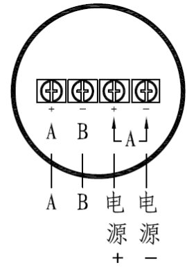
RS485输出
