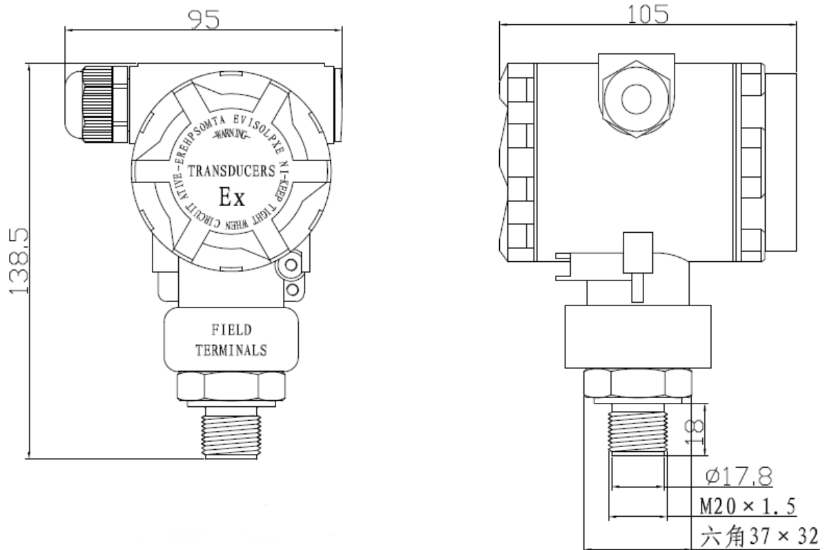
图二：外形参考图
