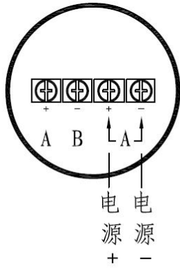
两线制电流输出
