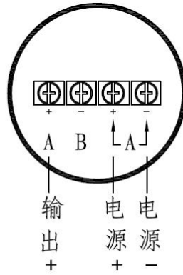
三线制电压/电流输出
