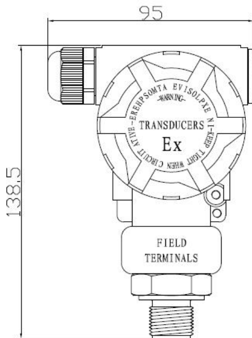
图二：外形参考图
